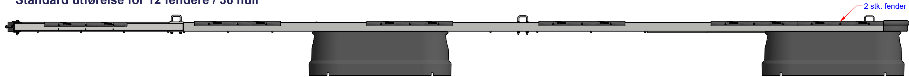
10 meter Standard utførelse for 12 fendere / 36 hull
