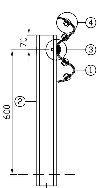
SNITT A:A
