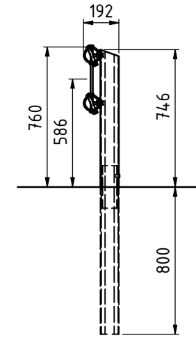
A-A ( 1 : 20 )
