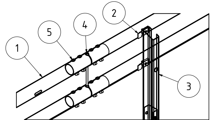
A-A ( 1 : 20 )
