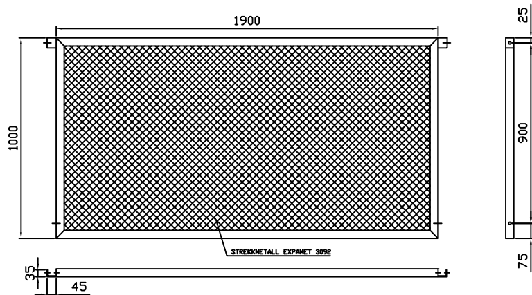
65290 Ramme med strekkmetall
