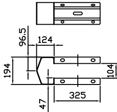
65056 Boksehanske for skinne 155, dobbel
