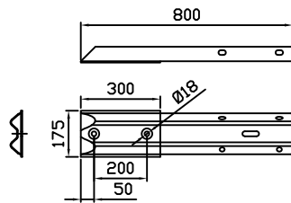
65053 Overgang for skinne 155 til betong
