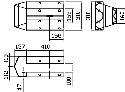
65057 Boksehanske for skinne 310/155
