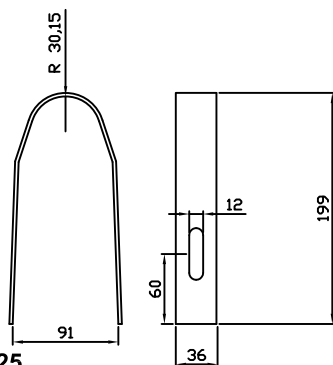
65325 Klammer for 2" for til Sigmastolpe
