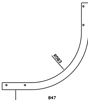
60102 Endestykke bøyd 90 L=1,3m
