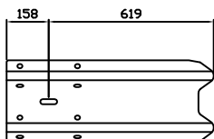
60055 Nedføring over 8 m universal skinne 310
