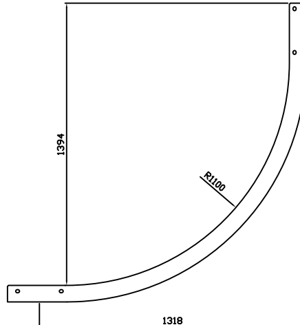
60106 Endestykke bøyd 90 L=2m
