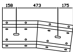
60055 Nedføring over 8 m universal skinne 310
