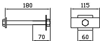
60601 Festesats for trestolp M16x180
