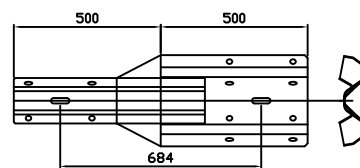
60159 Overg. skinne 310 til skinne 155
