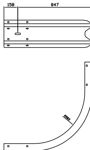
60143 Hjørne utv. 90 skinne 310 L=1,28 m
