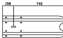
60050 Nedføring over 4 m universal skinne 310
