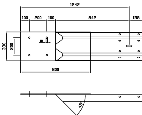
60151 Overgang fra skinne 310 til betong venstre 60150 Overgang fra skinne 310 til betong høyre
