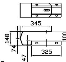
65055 Boksehanske for skinne 155, enkel
