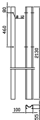
65200 Sigmastolpe 4 mm, L=2,13 m Ø12
