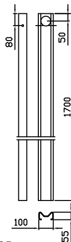
65205 Sigmastolpe 4 mm, L=1,7 m Ø12, endestolpe
