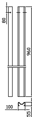
65245 Sigmastolpe 4 mm, L=0,96 m Ø12
