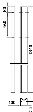
65215 Sigmastolpe 4 mm, L=1,34 m Ø12
